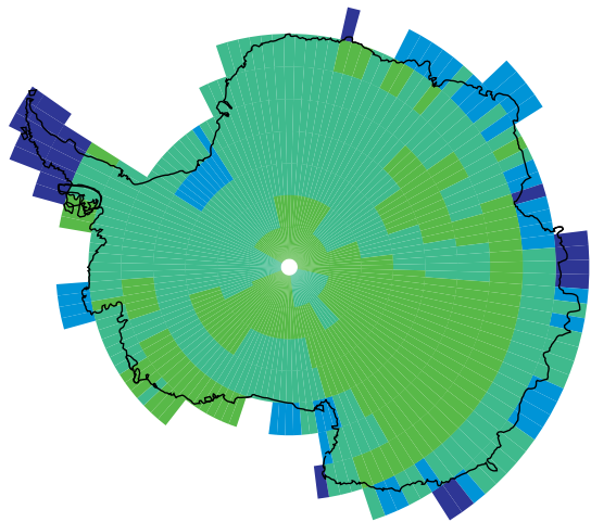
Mean % change in LGM2 relative to MET (total)
